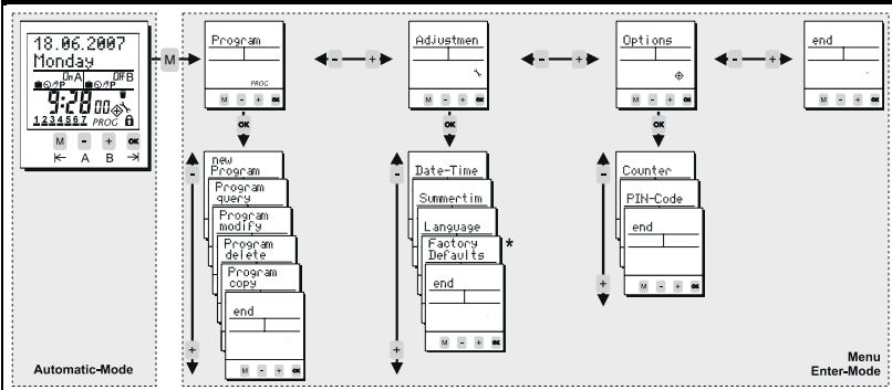
Automatic-Mode / Автоматический режим Menu / Меню Enter-Mode / Доступ к программированию
